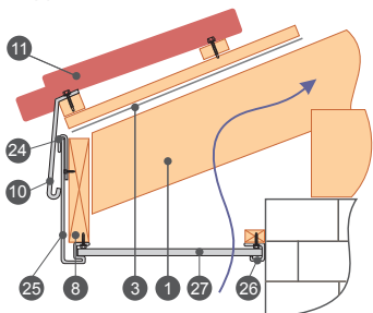
Подшивка свеса
